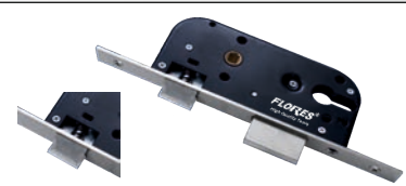
Broasca fara rulment pe butuc
